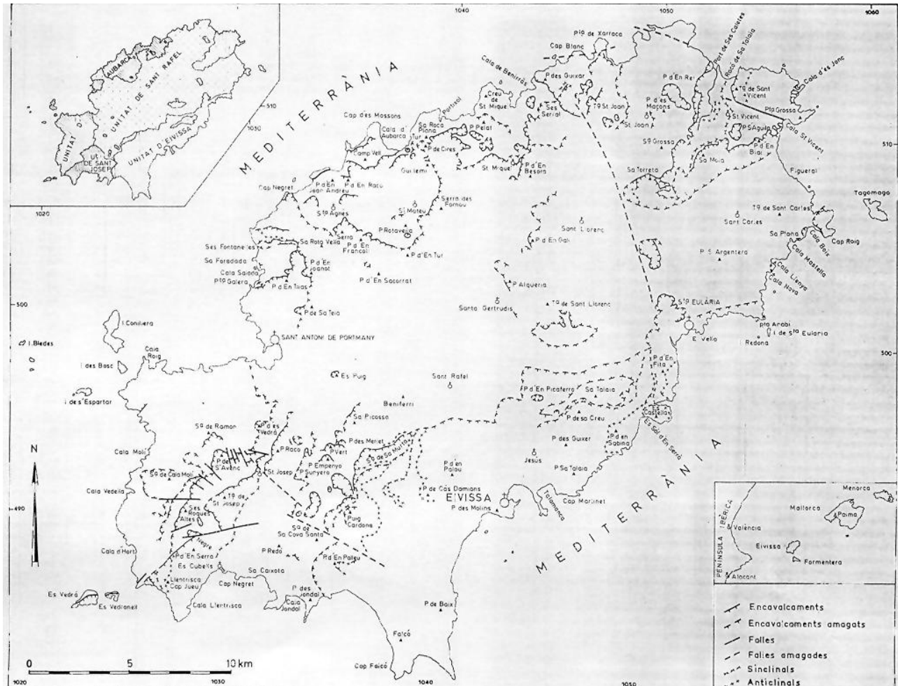
CARTA TECTÒNICA DE L'ILLA D'EIVISSA
